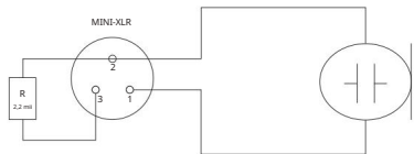
Condensator fără rezistență internă.
