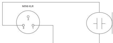
Condensator cu rezistență internă.
