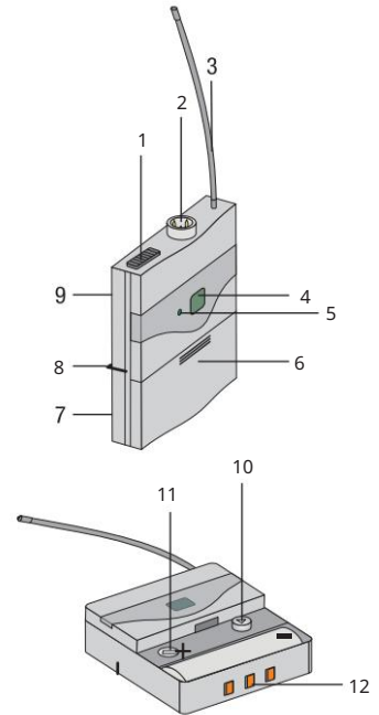
Figura 4: Comenzile Emițătorului PT420
