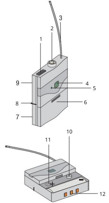
Figura 4: Comenzi pe transmițătorul PT420
