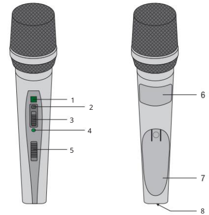
Figura 3: Dispozitive de control ale transmițătorului HT420
