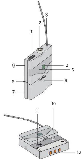
Figura 4: Comenzile transmițătorului PT420
