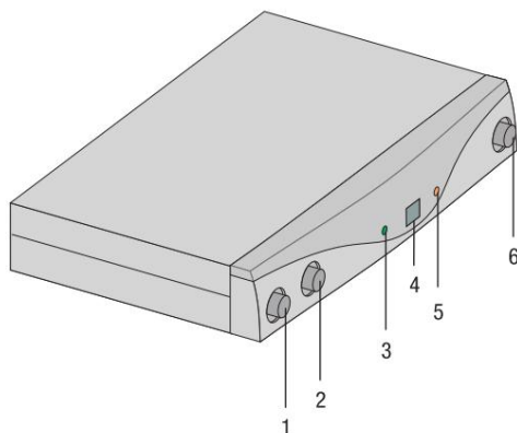
Figura 1: Elemente de control ale panoului frontal al receptorului SR 45
